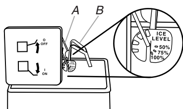
A. Wire shutoff arm
