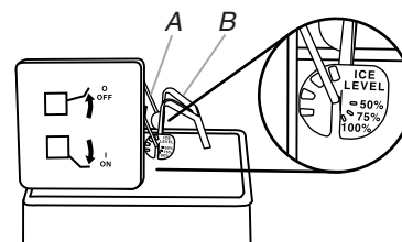
A. Bras de commande en broche B. Bras de réglage du niveau de glace
